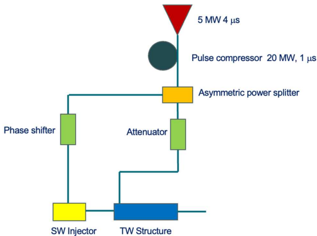
Figura 1 Schema a blocchi del sistema da progettare
